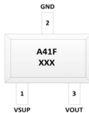
SOT23-3L
